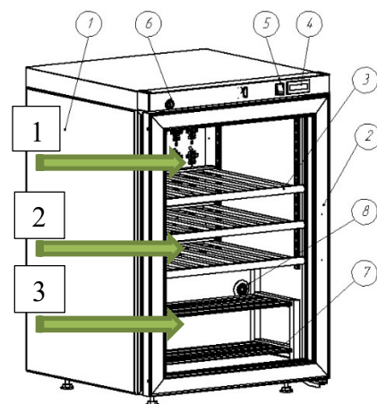
Рис.2. Внешний вид шкафа DW102-Bravo.
